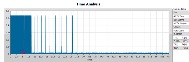
802.11a - 5500MHz (AWGN)
