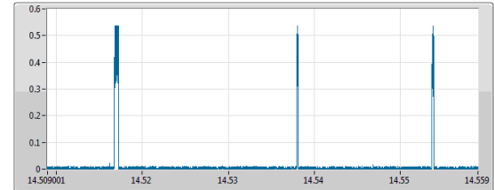
802.11a - 5500MHz (LTE)
