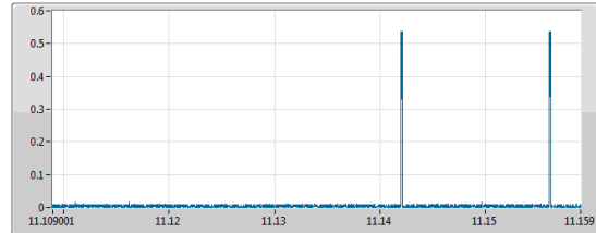
802.11a - 5500MHz (OFDM)
