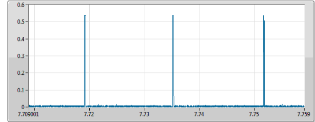
802.11a - 5180MHz (OFDM)
